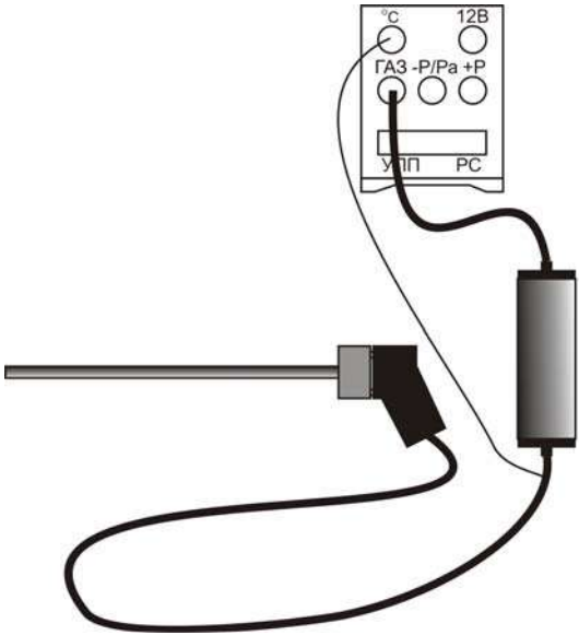
Рис. Б.3. Режим газоанализатор
