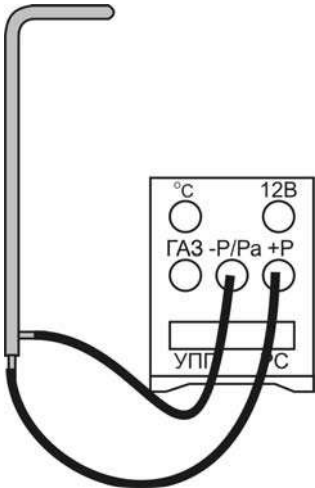
Рис. Б.5 Режим давление/скорость
